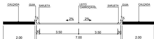
SEÇÃO TIPO II - Conforme Anexo C
