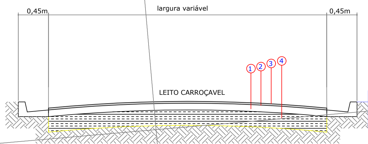
DETALHE CONSTRUTIVO PAVIMENTO ASFÁLTICO sem escala
