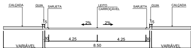
SEÇÃO TIPO I - Conforme Anexo C
