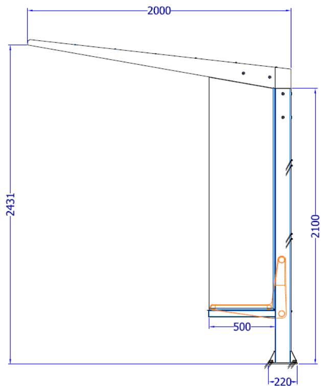
ABRIGO 2,00 X 3,00m - VISTA LATERAL
