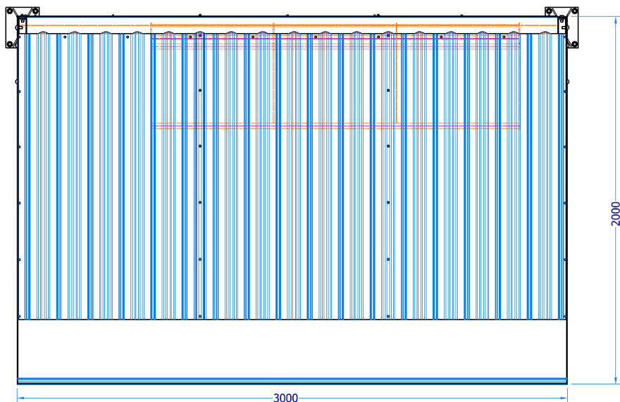
ABRIGO 2,00 X 3,00m - VISTO DE CIMA
